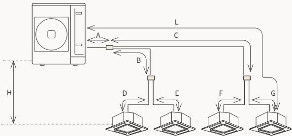
Configuración 4x1 (de 4 a 6 CV)
