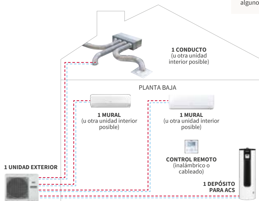
Ejemplo instalación
