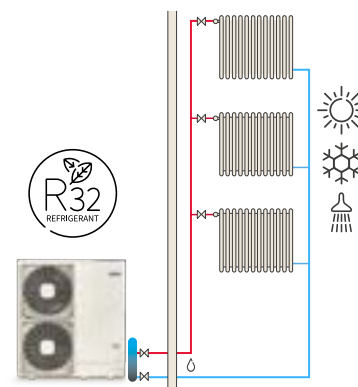
Unidad exterior R32 Intercambiador R32/ H2O
