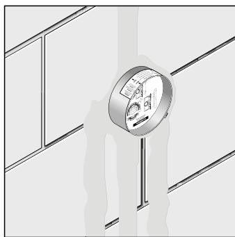
Instalación directa en la pared
