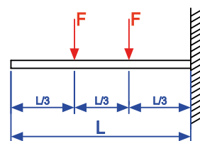
Dos cargas puntuales en L/3
