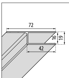
A PARED perfil de la pared lateral todos los modelos
