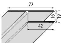
FREE 2 H 85 cm
