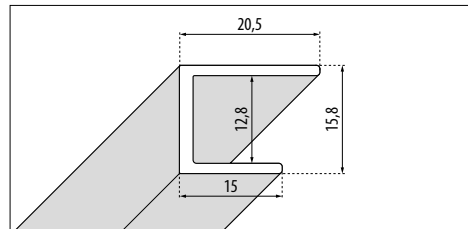
A PARED N180 1B - lado del magneto
