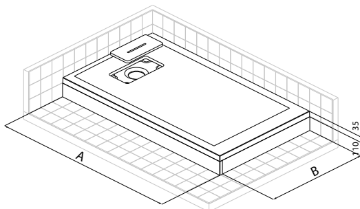
INSTALACIÓN OPCIONAL CON PIES REGULABLES Y PANEL AJUSTABLE A MEDIDA. INSTALAÇÃO OPCIONAL COM PES REGULAVEIS E PAINEL AJUSTAVEL A MEDIDA.
