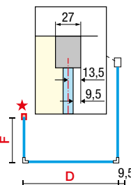
Pieza de sujeción del cristal a suelo Peça de fixação do vidro ao chão
