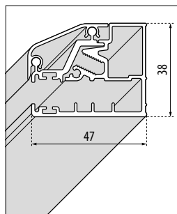
A PARED para fijo lateral
