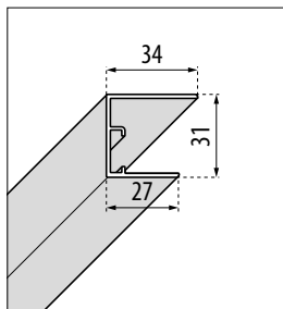
A PARED para todos los modelos
