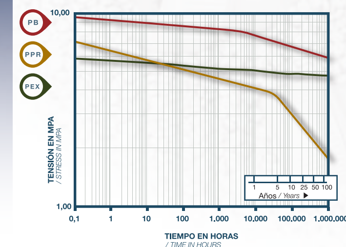
CURVAS DE REGRESIÓN DE VARIOS MATERIALES A 80°C / REGRESSION CURVES OF SEVERAL MATERIALS AT 80°C
