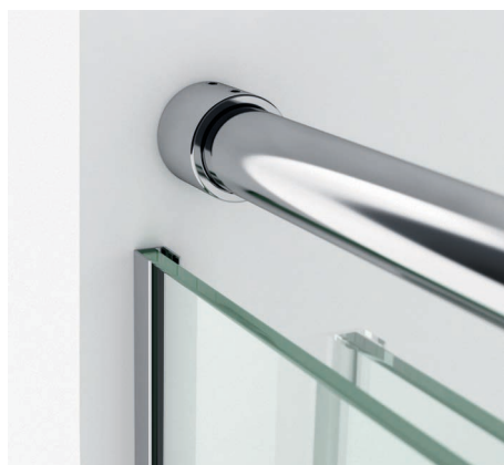
04 Fijación de la guía superior y del elemento fijo (con perfil en forma de "u" en acero inoxidable) a la pared.
