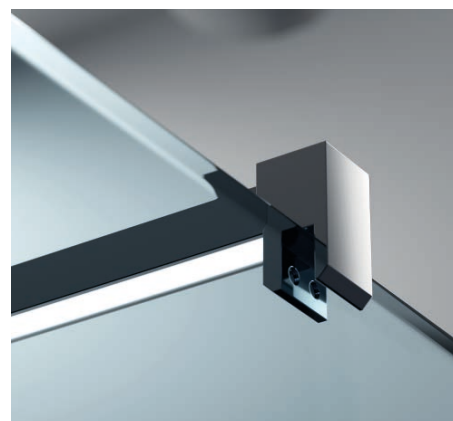
07 Detalle de la pinza de sujeción de la barra (con iluminación LED) al fijo en acero inoxidable.
