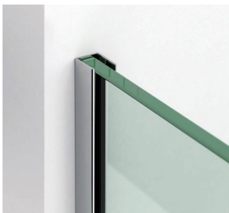
03 Fijación del elemento fijo a la pared con perfil en forma de "u".
