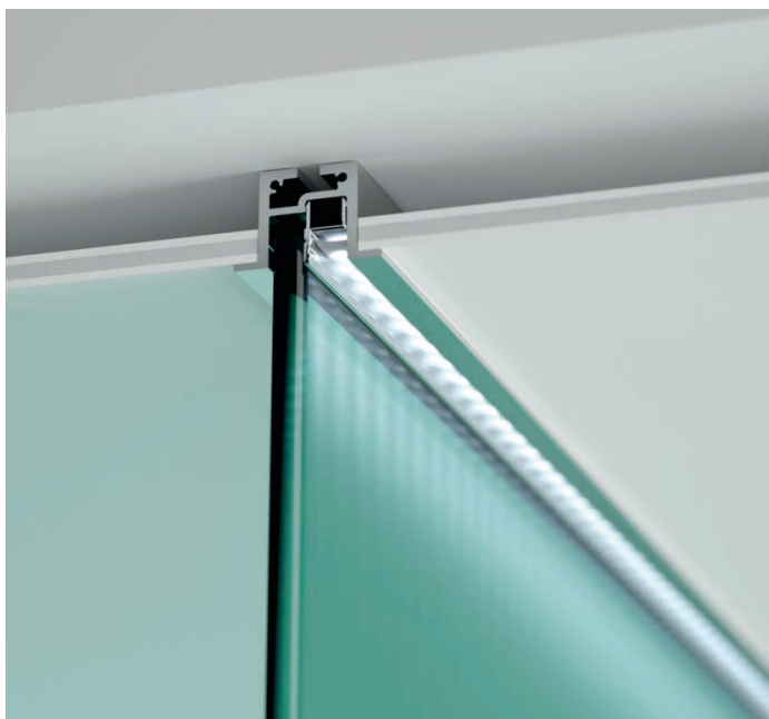
01 Perfil superior para sujetar el cristal fijo, iluminado con leds.
