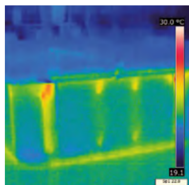
Test de fugas de calor realizado con el sistema Nordic Insulation System
