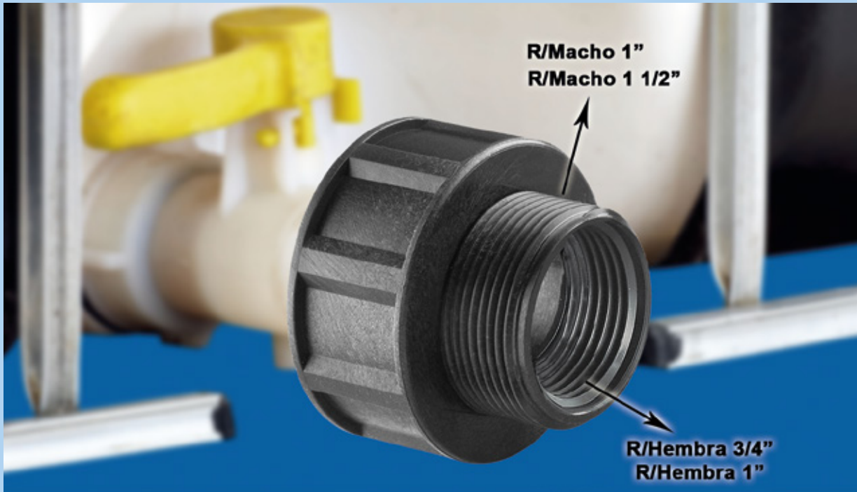
ADAPTATEUR UNIVERSEL POUR CUVES ADAPTADOR MACHO-HEMBRA UNIV. BIDAO
